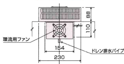
【冷却側正面図】
