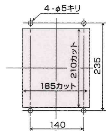
【筐体カット及び取付穴】
