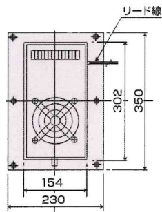
【タテ型冷却側正面図】
