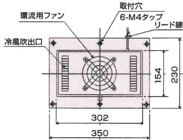
【冷却側正面図】
