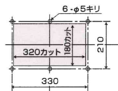
【仕様】(PFC採用電源) Standard
