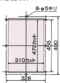
【筐体カット及び取付穴】
