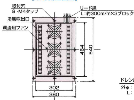
【冷却側正面図】
