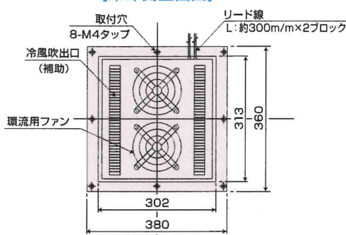
【冷却側正面図】
