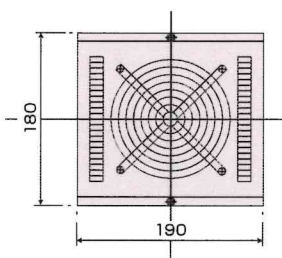
【放熱側正面図】
