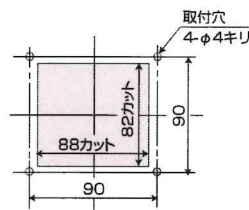
【筐体カット及び取付穴】
