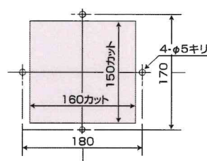
【筐体カット及び取付穴】
