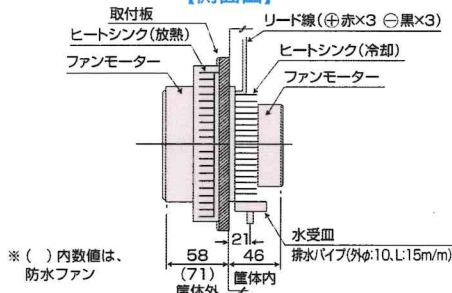
【側面図】
